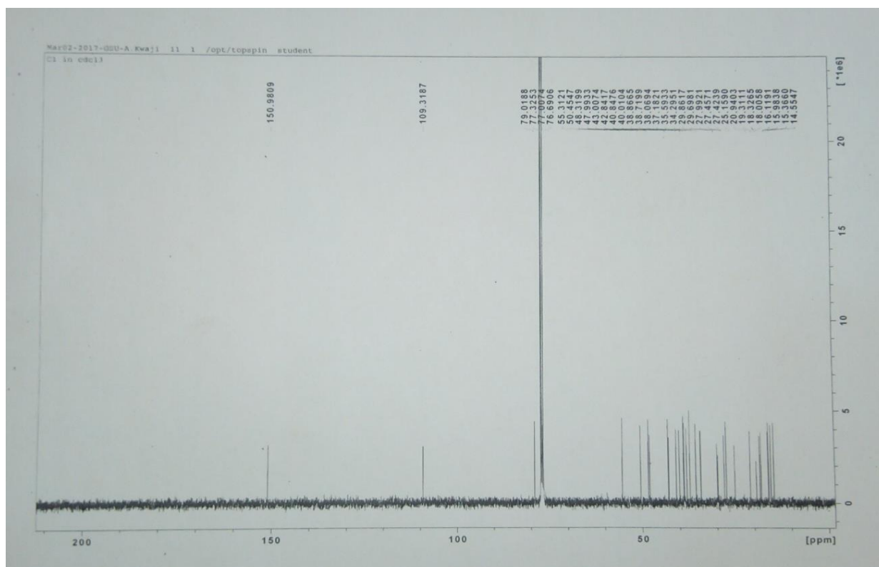
13 C-NMR Spectrum of Enac1
